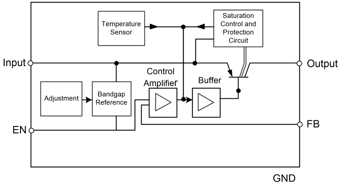
图 4-2 BST6008LADJ 模块框图
