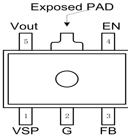
图3-2 BST6008LADJ管脚配置图
