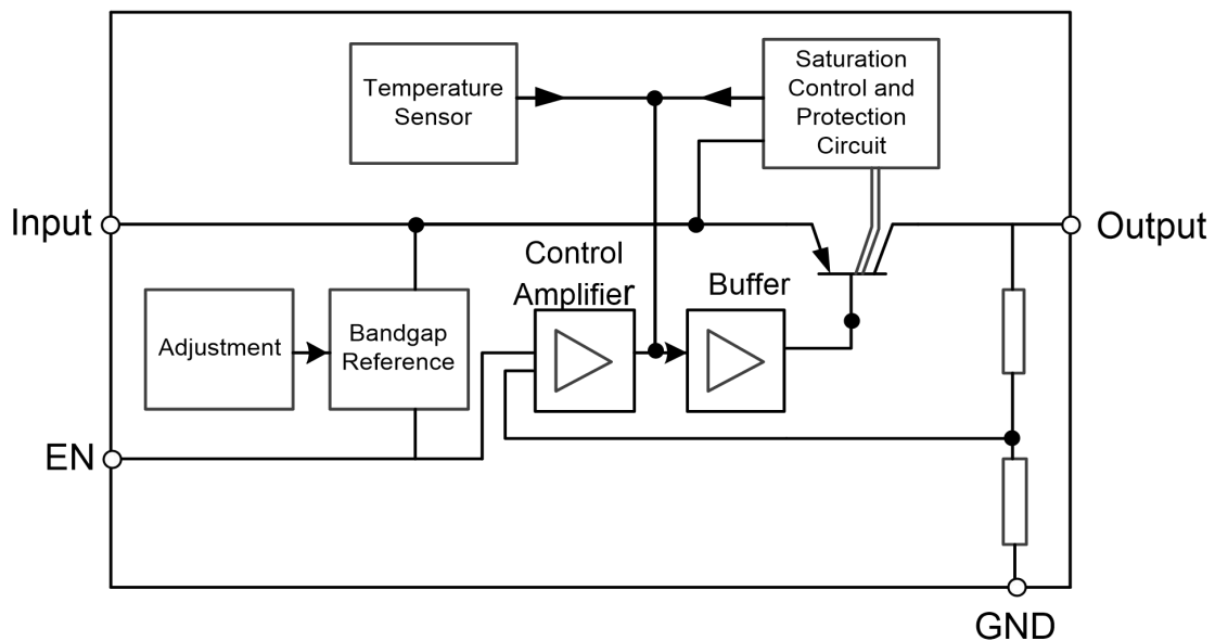
图 4-1 BST6008L33/L50 模块框图
